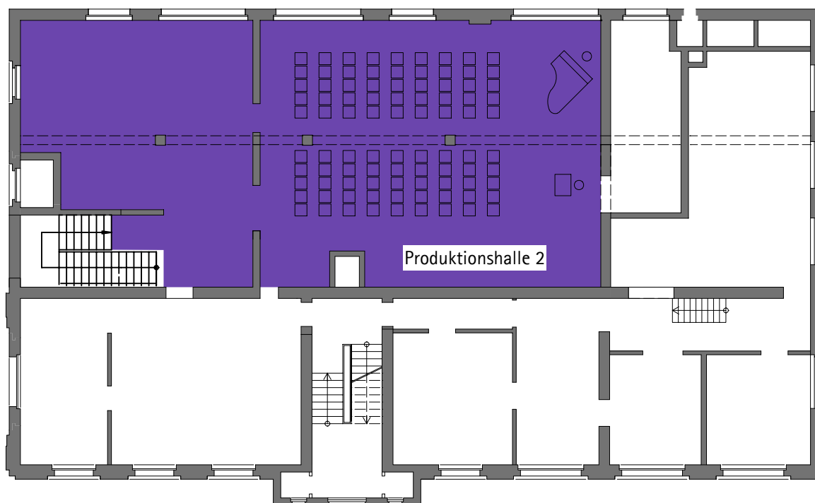
1. Obergeschoss
